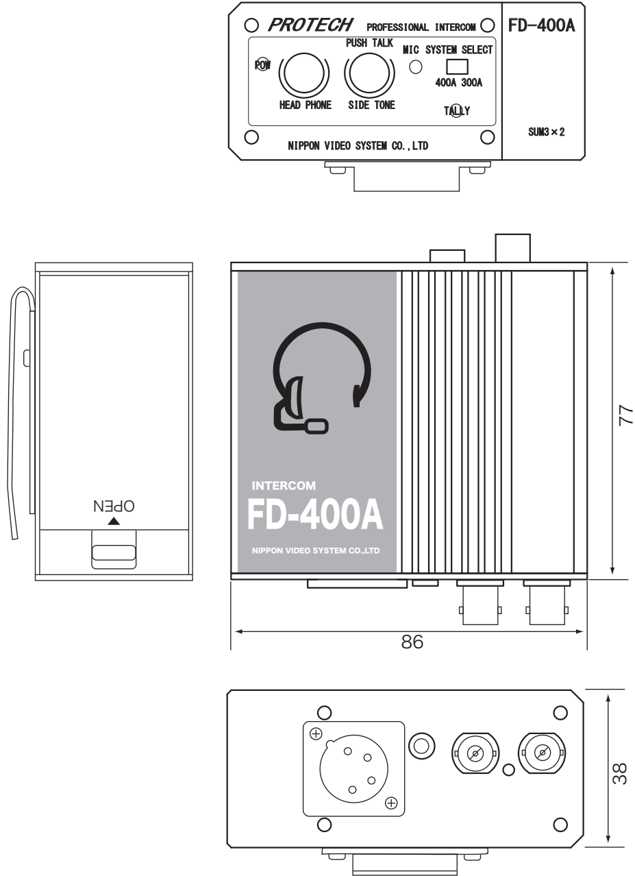
外形寸法図 (単位 : mm) Dimensions (unit: mm)
