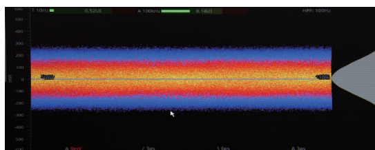
信号が衰下した状態のアイパターン
