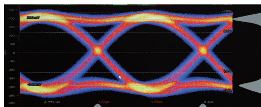
プロテック VHD シリーズ使用時のアイパターン
