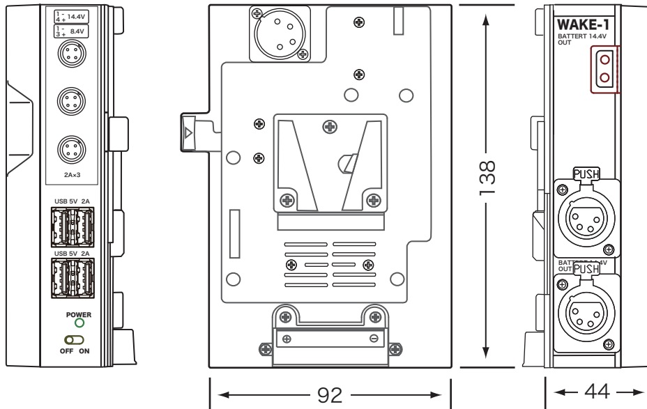
Vマウントバッテリーホルダー <DC入力> (Vマウントバッテリー装着) (REAR)(バッテリー側)
