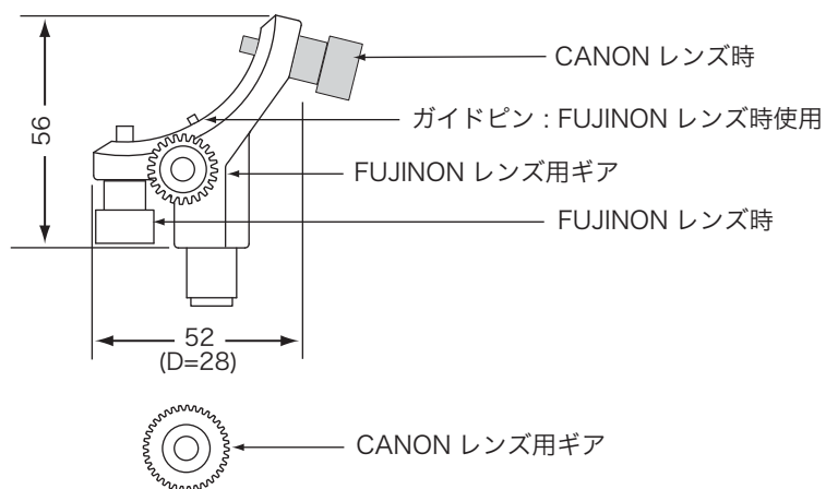
ユニバーサルシャフト
