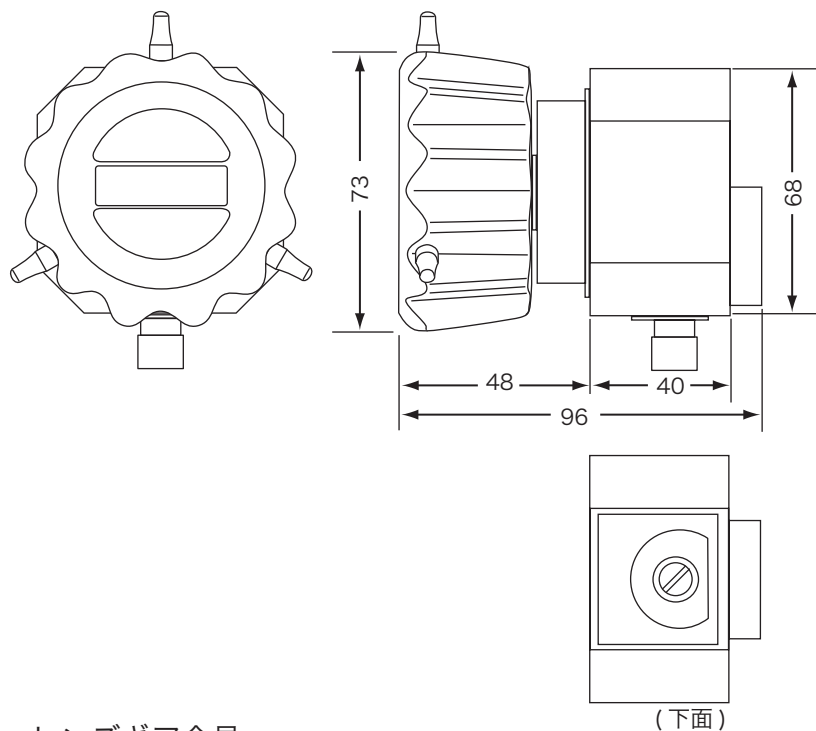
レンズギア金具
