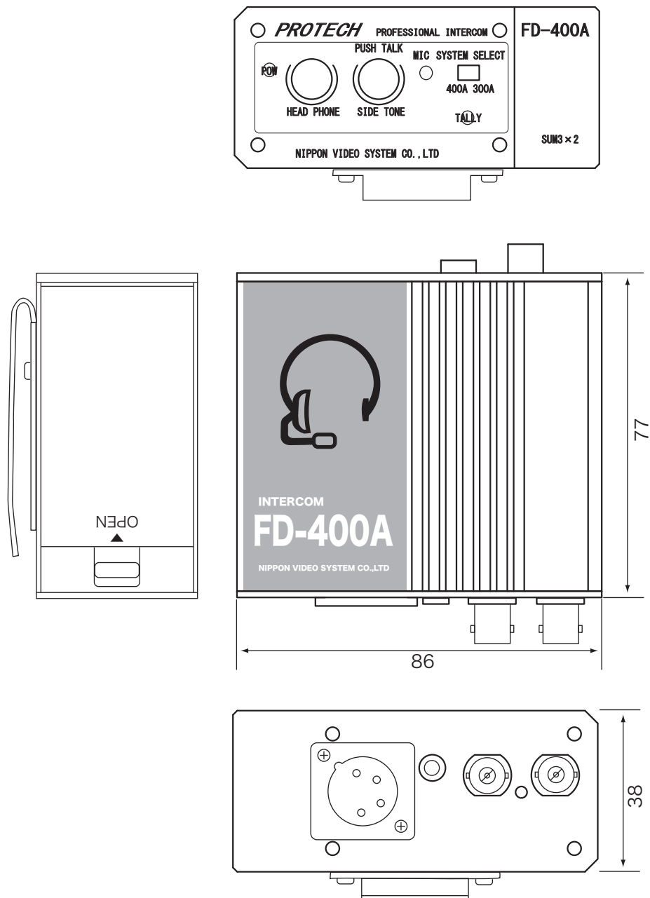
外形寸法図(単位:ミリ) Outside dimension (unit: mm)
